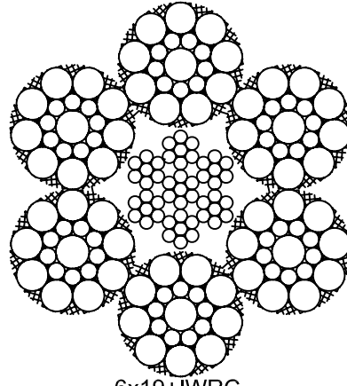
6x19+IWRC
