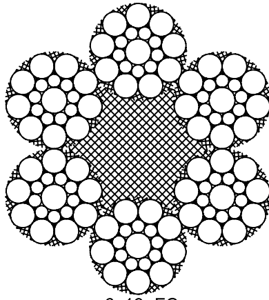
6x19+FC
