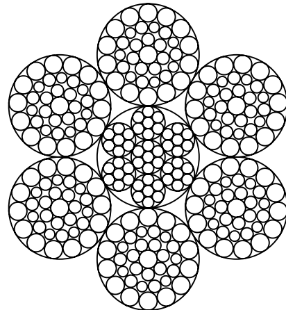
6x36WS+IWRC
