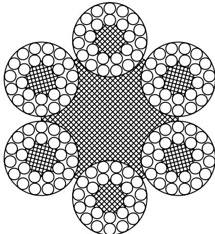
6x24+7FC
