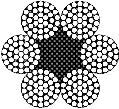
6x37+FC
