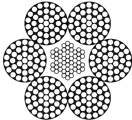
6x37+IWRC
