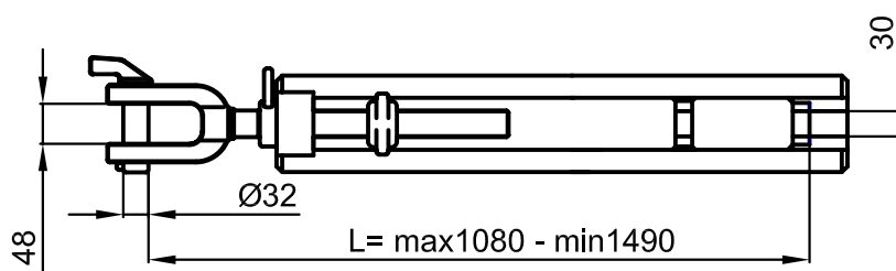
Jaw - knob type B-31
